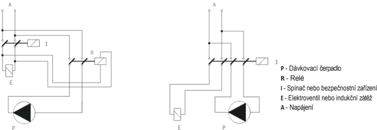
Obr. 10. Elektrická instalace.
