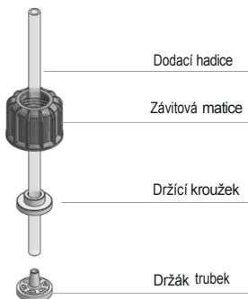
Obr. 7. Montáž přívodní hadice / hlavy čerpadla
