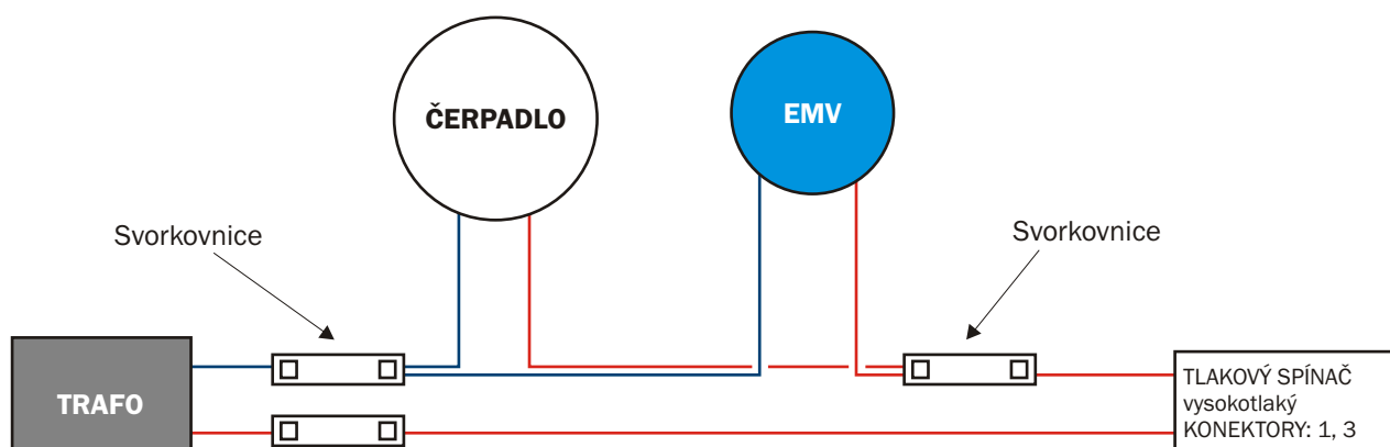
Standardní zapojení - jeden tlakový spínač
